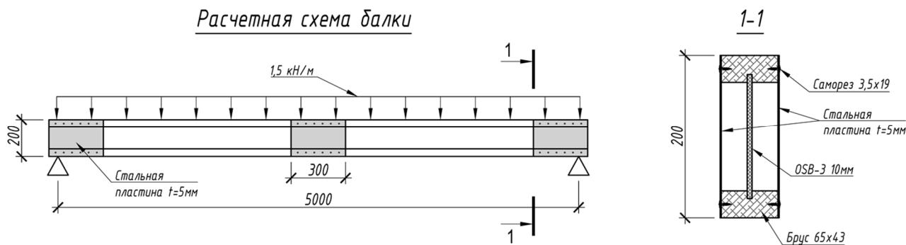
Рис. 1. Расчетная схема двутавровой балки
