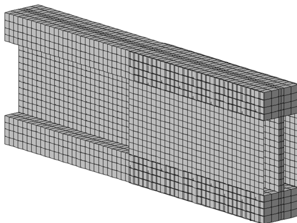
Рис. 2. Фрагмент расчетной модели (опорный участок балки)
